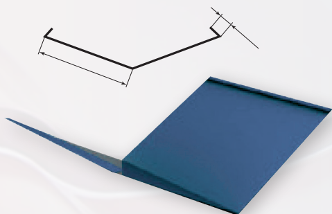
RYNNA KOSZOWA (wymiary wg zamówienia)
