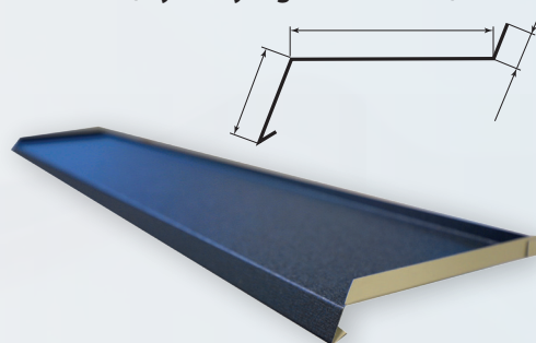
PARAPET (wymiary wg zamówienia)
